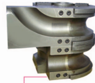
直徑模 (拉彎) (Bending Die/Draw Bending)
