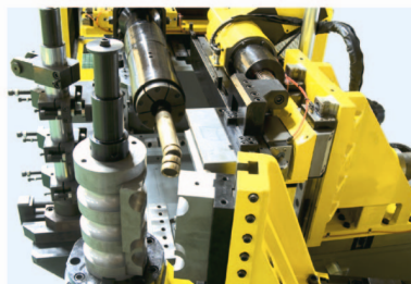
車頭特寫 Bending Head
