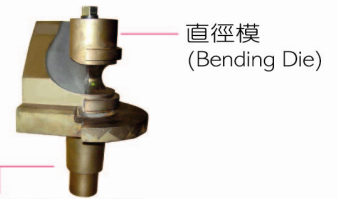
直徑模 (拉彎) (Bending Die/Draw Bending)
