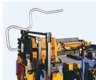
多層模車頭特寫 Multi-Levels
