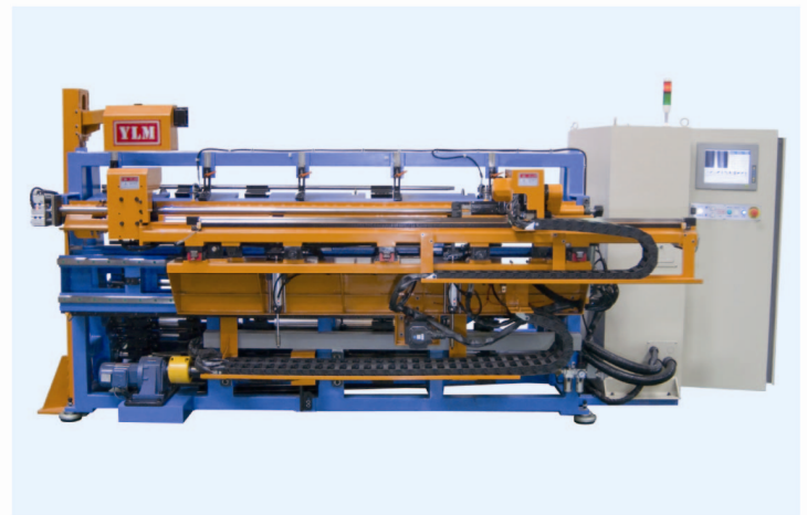
自動餵料焊道偵測 Weld seam detection
