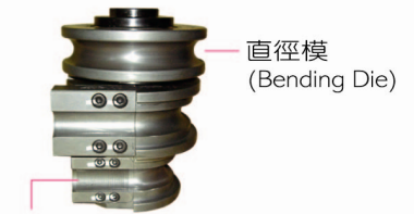
直徑模 (拉彎) (Bending Die/Draw Bending)
