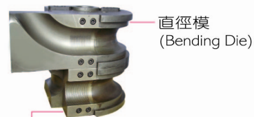
直徑模(拉彎) (Bending Die/Draw Bending)
